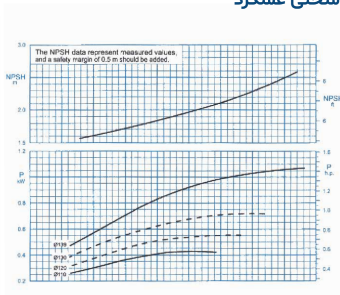
منحنی عملکرد
